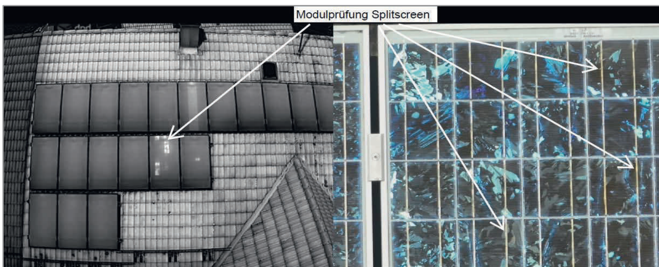
Überflug über Photovoltaikanlage Detailanalyse mittels Splitscreen (Wärmebildkamera / 56-facher Hybridzoomkamera) Ersehtlich: Defekt durch verfärbte / korrodierte Leiter im Modul
