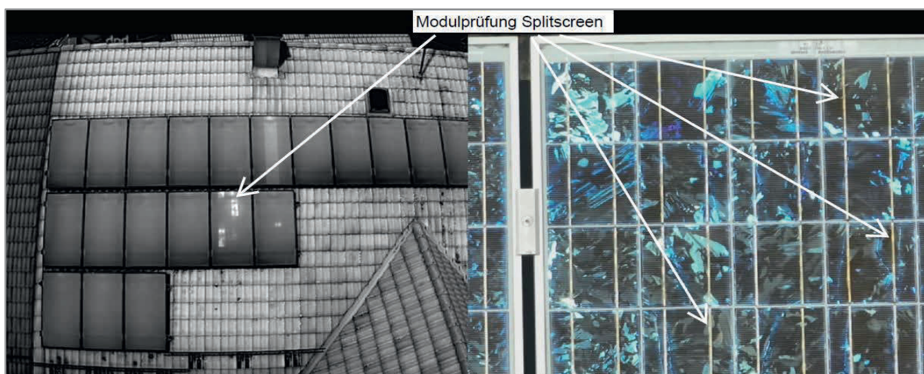
Überflug über Photovoltaikanlage Detailanalyse mittels Splitscreen (Wärmebildkamera / 56-facher Hybridzoomkamera) Ersichtlich: Defekt durch verfärbte / korrodierte Leiter im Modul
