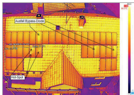
Überflug über Photovoltaikanlage Hotspotauswertung mittels Wärmebildkamera & Thermografiesoftware
